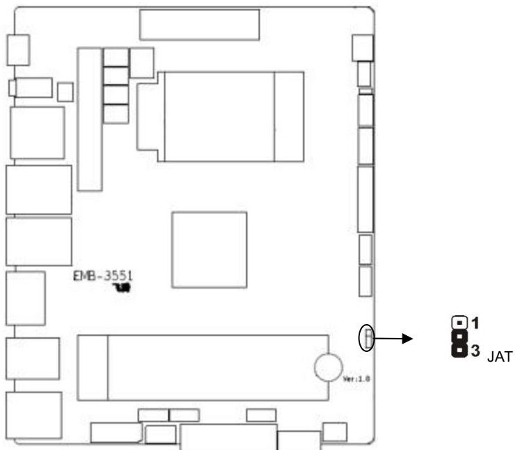
JAT：上电自启和非上电自启选择（默认上电自启）
