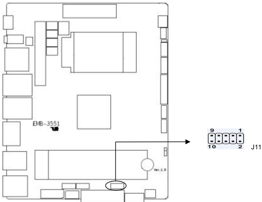
J11: LVDS 电压选择
