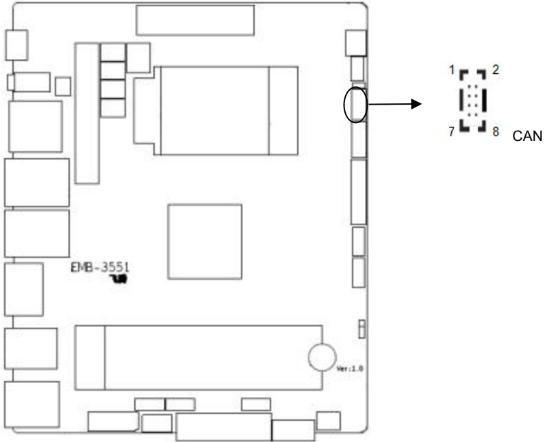
CAN 接口：2X4PIN 2.0mm 小白座
