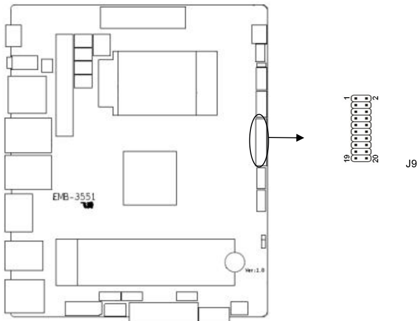
J9: 2X10PIN 2.0mm 小白座, 信号电平全部为 3.3V
