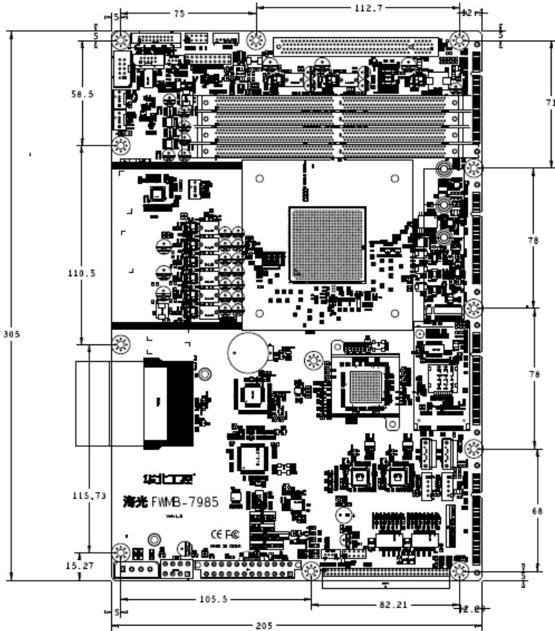
FWMB-7985 接口位置和尺寸图
