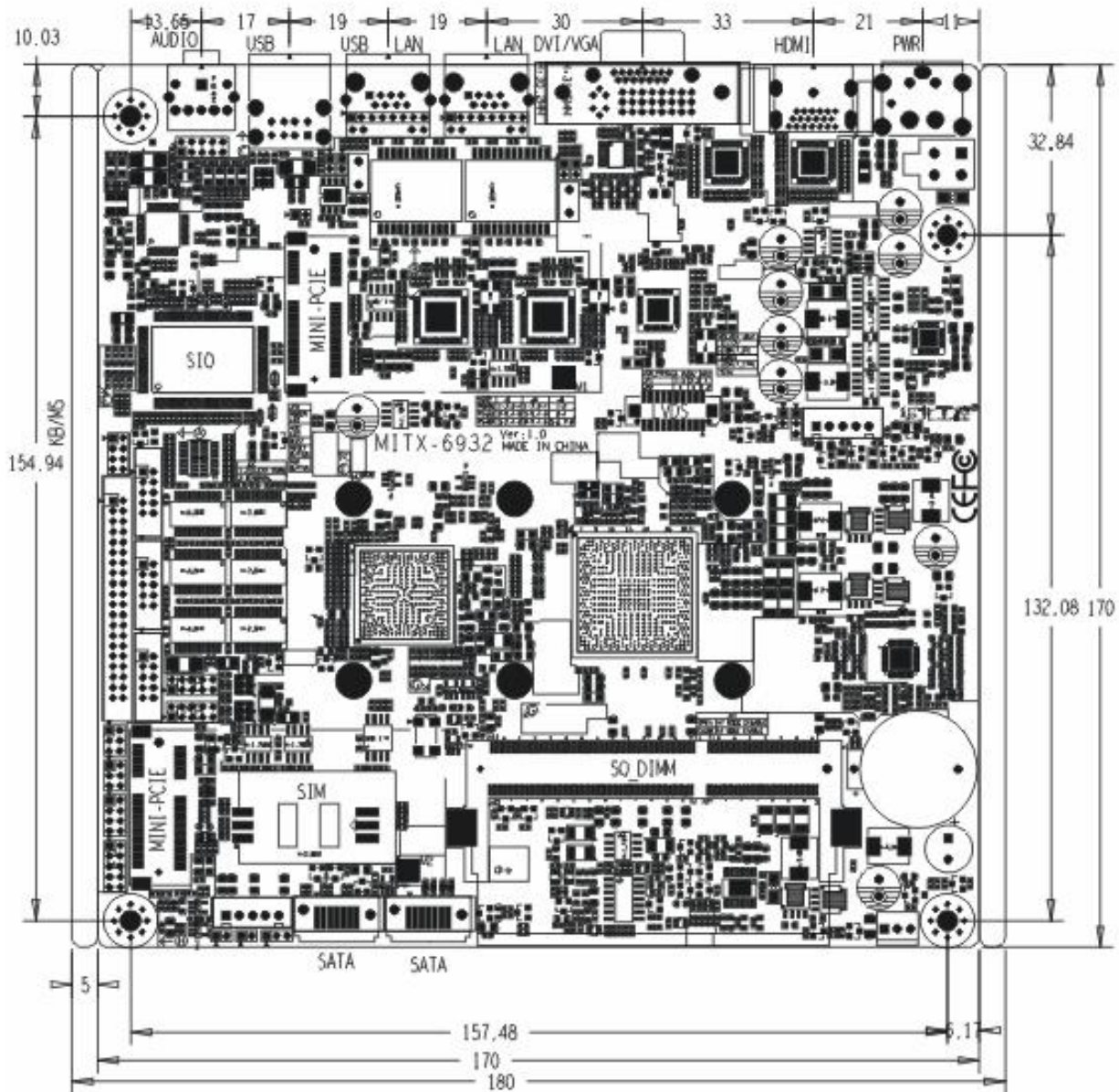
MITX-6932 接口位置和尺寸图
