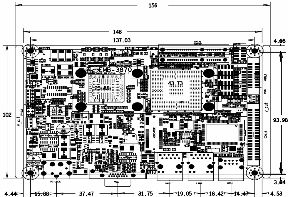
EMB-3870 尺寸和接口位置图
